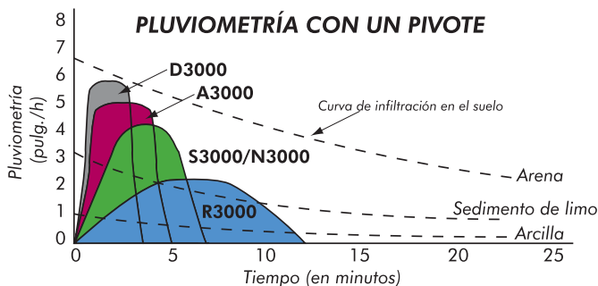
Curvas de infiltración típicas combinadas a la pluviometría del pivote (al final de un sistema de 1/4 milla - 400m - con un caudal de 8 GPM/Acre - 4,5 m 3 /hr/ha - y una velocidad de traslado de 5 fpm. - 1,5/min.)
